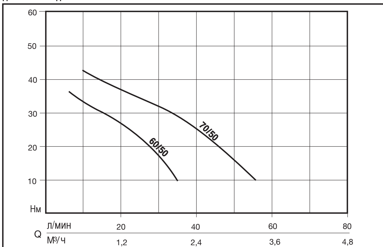
ДИАГРАММА ГИДРАВЛИЧЕСКИХ ХАРАКТЕРИСТИК
