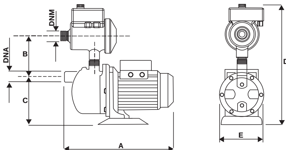
ГАБАРИТНЫЕ РАЗМЕРЫ И ВЕС
