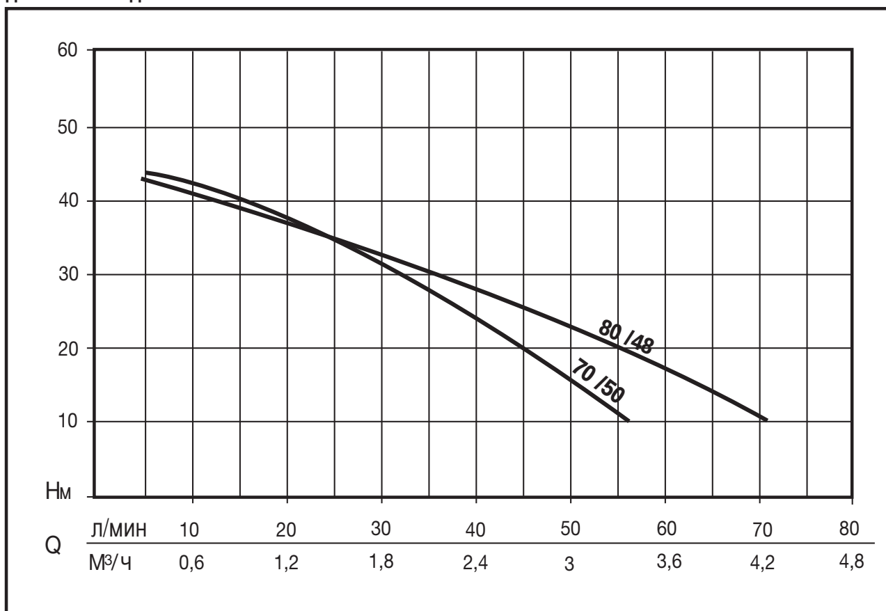
ДИАГРАММА ГИДРАВЛИЧЕСКИХ ХАРАКТЕРИСТИК
