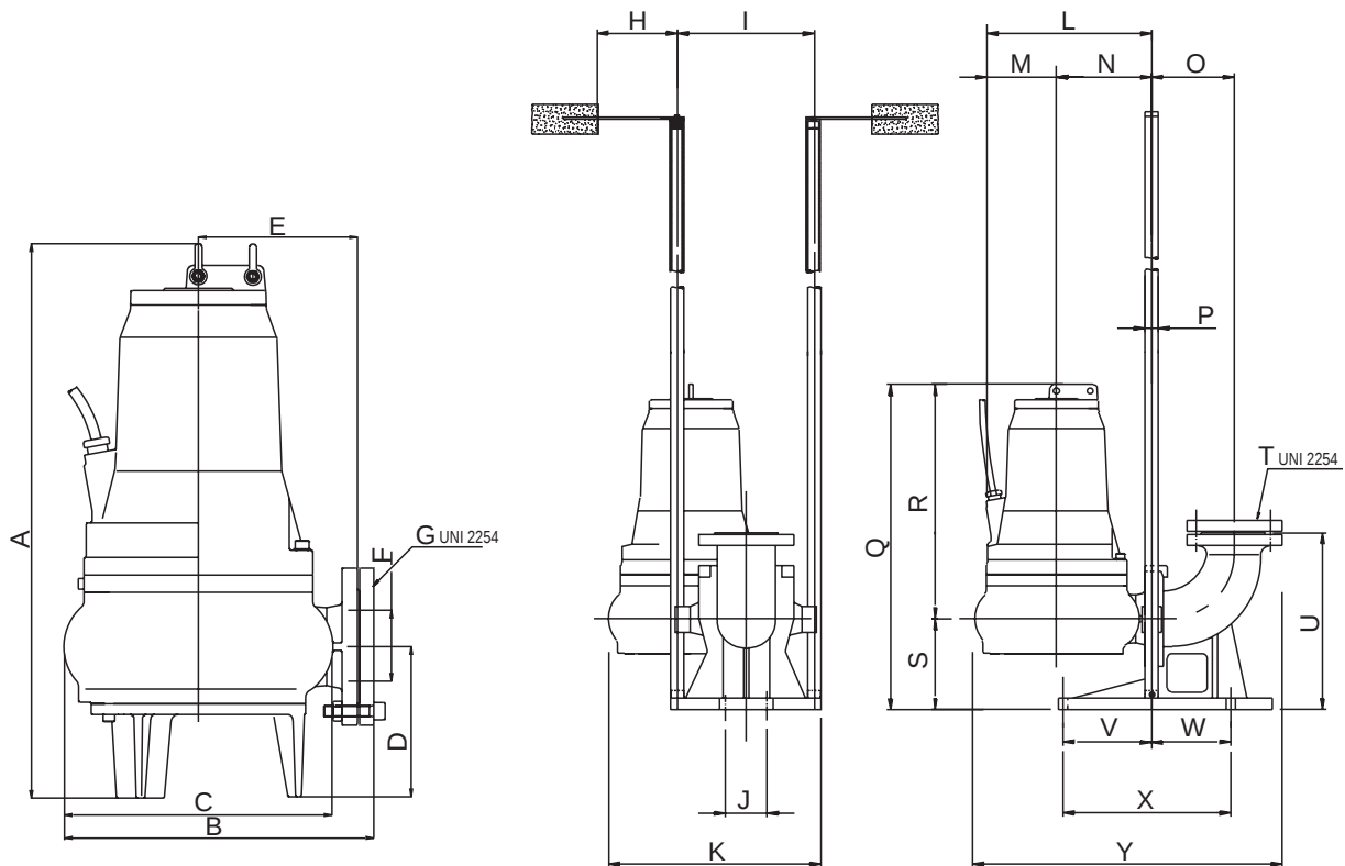
ГАБАРИТНЫЕ РАЗМЕРЫ И ВЕС
