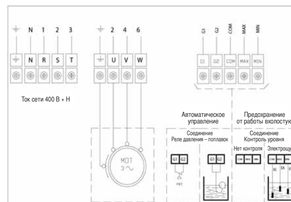
Схема подключения
